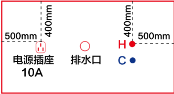
独立缸水电图
